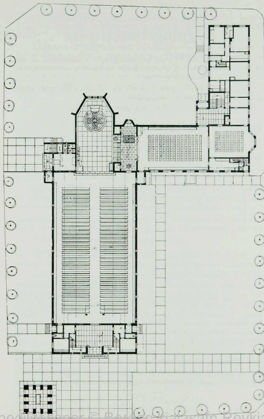
Plan av kirken i mål 1 : 500.
